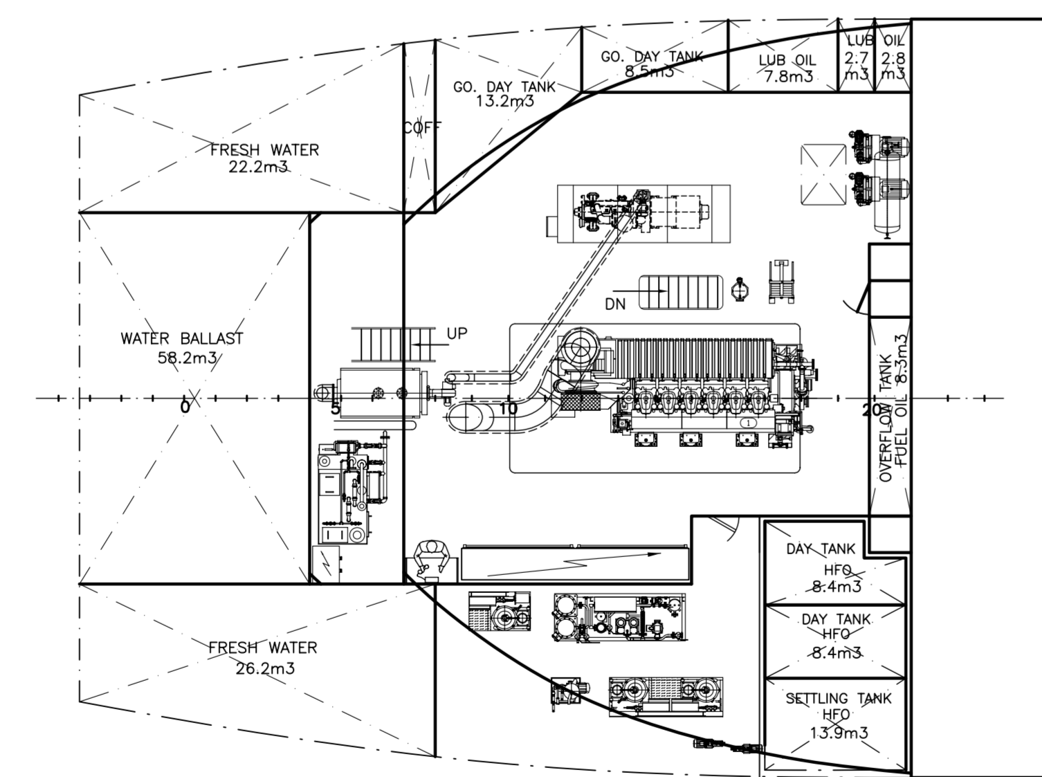
UPPER ER DECK
