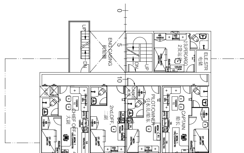
C甲板 C DECK 22150
