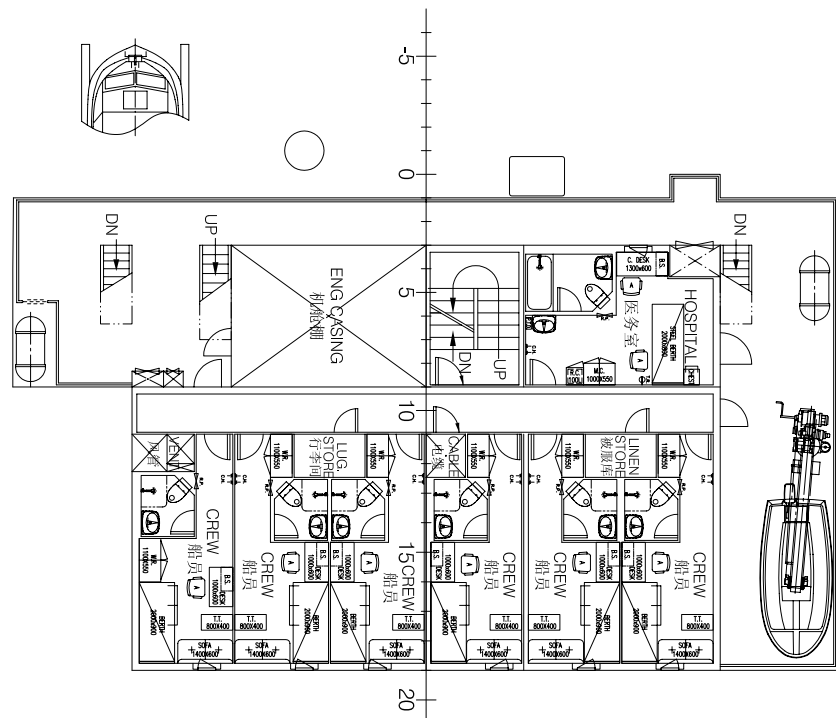
A甲板 A DECK 16760
