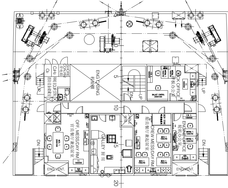
尾樓甲板 POOP DECK 14050
