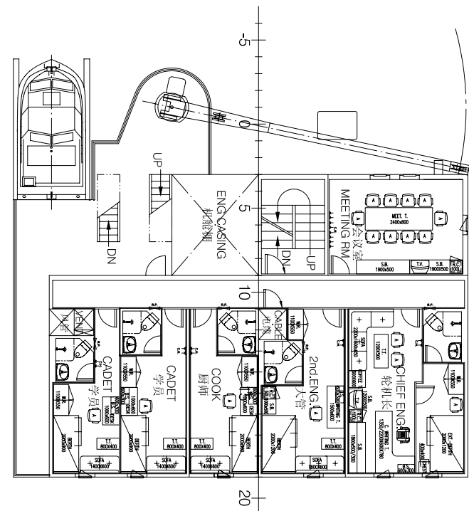
B甲板 B DECK 19450
